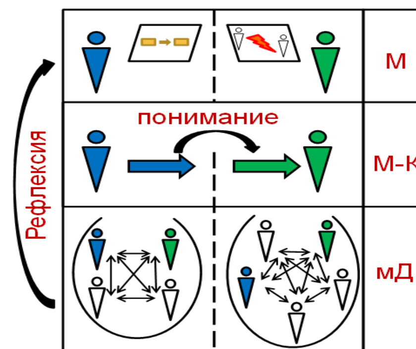
Схема мыследеятельности
