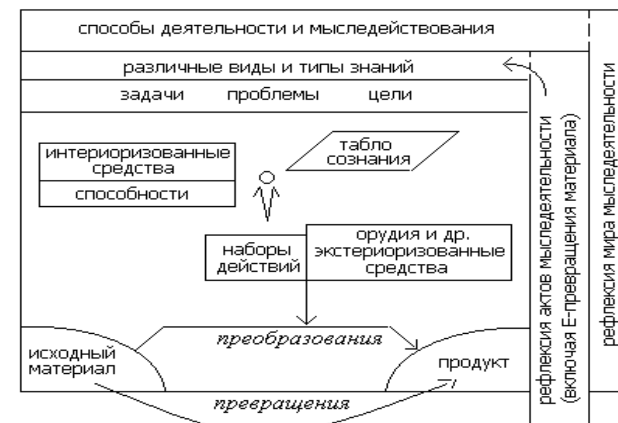
Схема мыследеятельности
